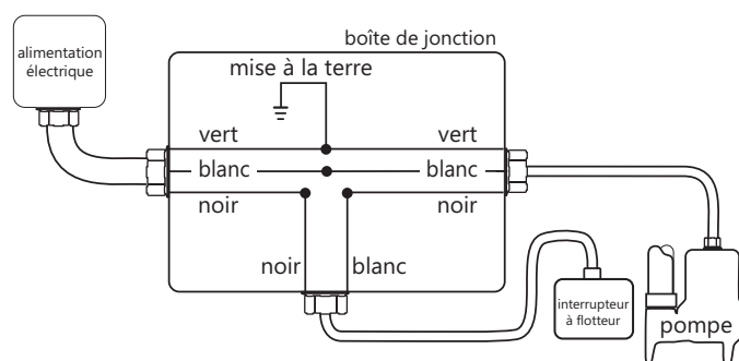
Figure 3. Câblage direct de pompes automatiques
