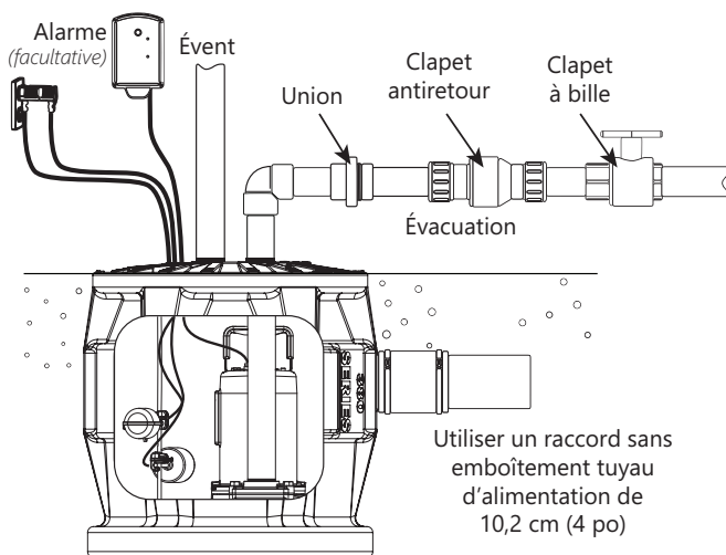
Figure 1. Installation intérieure typique (série Pro380 illustrée)
